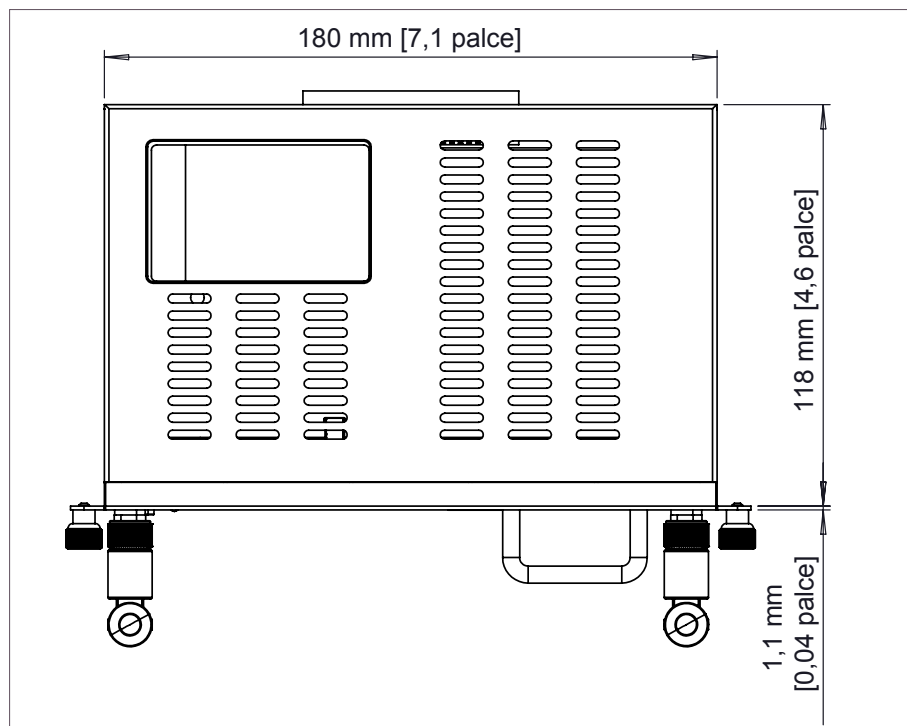
Pohled shora
